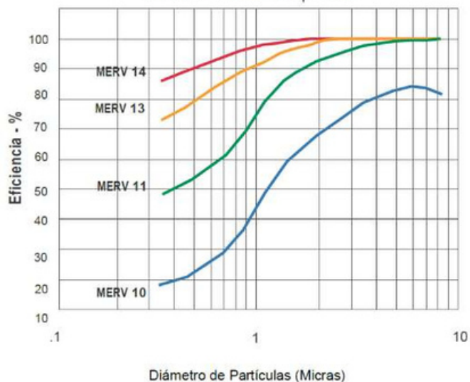
Eficiencia Mínima del Filtro Eficiencia vs. Tamaño de partícula
